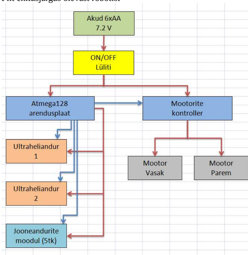
Elektriskeem
